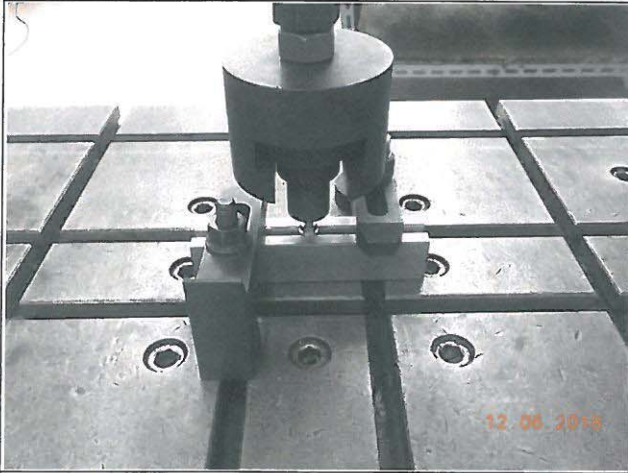
抗拉試驗 石中劍 T 型無縫鋼支架
