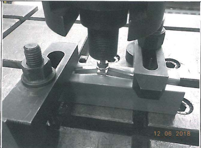
試驗後樣品 石中劍 T 型無縫鋼支架
